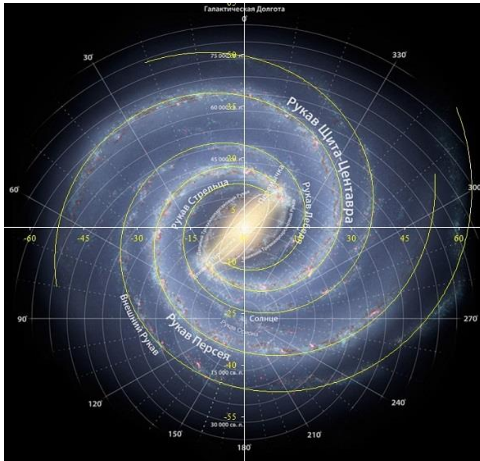
Рис.1 Карта галактики Млечный Путь [1] с нанесёнными на неё функциональными кривыми, аппроксимирующими форму рукавов.
