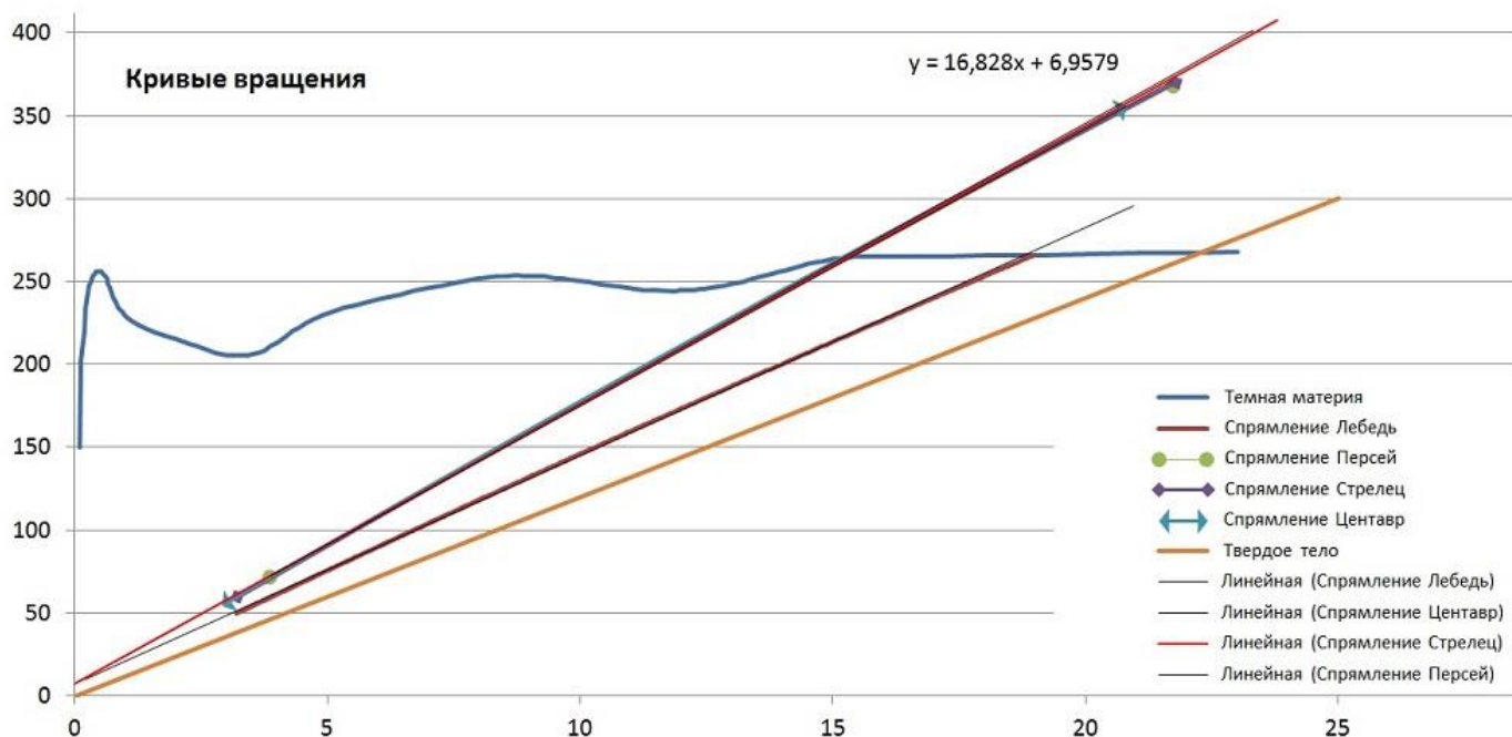
Рис.3 Кривые вращения – наблюдаемая и спрямляющие за 3 млрд. лет. Сверху уравнение линейного тренда спрямляющей кривой вращения Стрельца.
