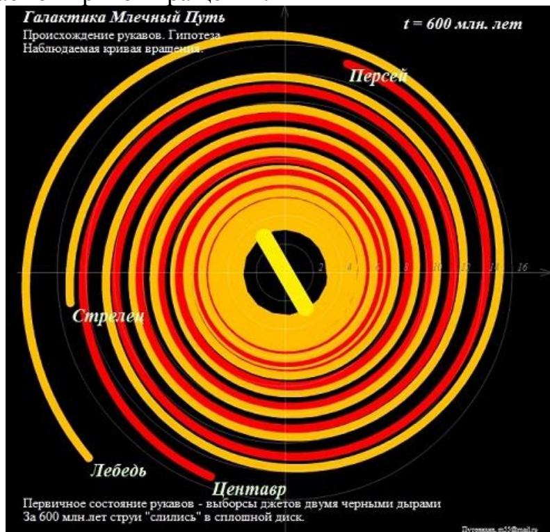
Рис.6 Модель галактики Млечный Путь с рукавами - джетами через 600 млн. лет после их образования и вращения с наблюдаемой кривой вращения
