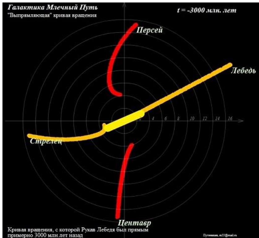
Рис.2 Так могла выглядеть галактика Млечный Путь 3000 млн. лет назад в результате коллапса двух звёзд и выброса ими двух пар джетов
