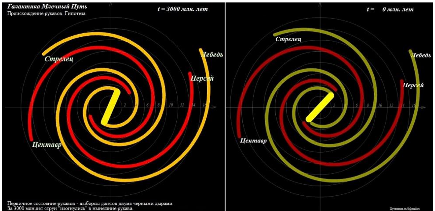
Рис.4 Изображение галактики Млечный Путь с рукавами, образованными за 3 млрд. лет из двух пар джетов (слева) и нынешнее её представление (справа). Кривая вращения – выпрямляющая Рукав Лебеда.
