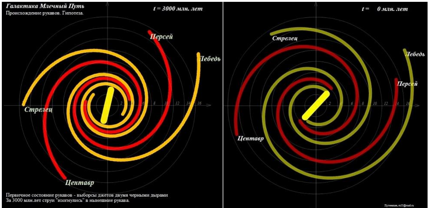
Рис.5 Изображение галактики Млечный Путь с рукавами, образованными за 3 млрд. лет из двух пар джетов (слева) и нынешнее её представление (справа). Кривая вращения – выпрямляющая Рукава Лебеда.
