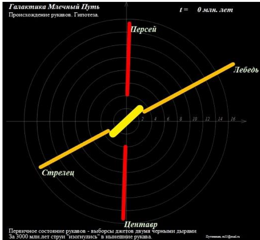
Рис.3 Вид рукавов галактики Млечный Путь в момент их возникновения
