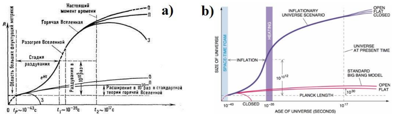
Рис.2. Согласно новым инфляционным теориям за время раздувания порядка 10^{-35} с Вселенная увеличивается по разным оценкам в 10^{100\,000} - 10^{1\,000\,000\,000\,000} раз. Рисунки из работ (слева направо) [12, 9]
