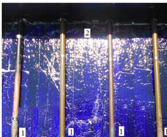
Рис.1.Крепление термосифонов в термостате.1.Термосифоны.2.Нагрузка термостата.
