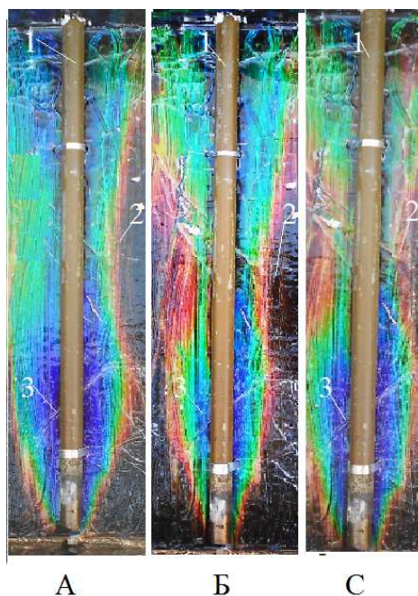
Рис.2.Внешние термограммы термосифонов. 1.зона конденсации.2.Транспортный канал.3.Зона парообразования.
