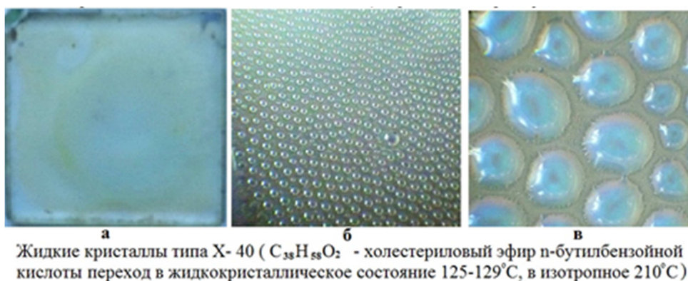
Рис.2.Динамика формирования текстуры жидкого кристалла X-40 в коронном разряде. а. Плоский электрод с плёнкой жидких кристаллов. б. Сетка из «застывших» оптических ячеек жидких кристаллов. в. Ячейки жидких кристаллов в электрическом поле.
