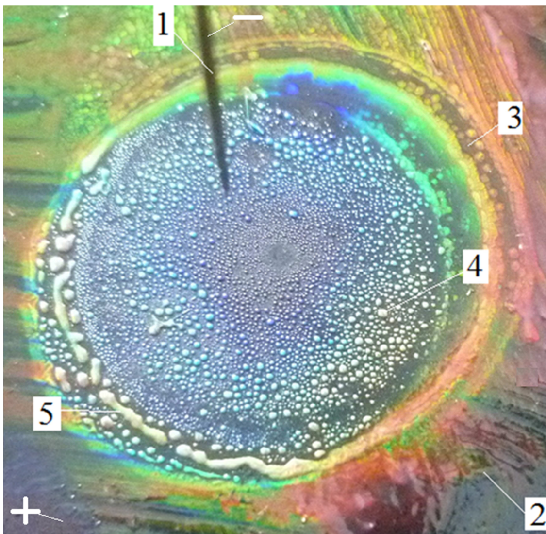
Рис.5. Плёнка ХЖК в неоднородном электрическом поле коронного разряда.1.Электрод типа игла. На игле отрицательный потенциал. 2.Проводящая стеклянная подложка или плоский металлический электрод.3. Граница коронарного отпечатка в плёнке жидких кристаллов.4.Возбуждённые, вращающиеся ячейки ХЖК типа Х-40. 5. Объединённые ячейки.
