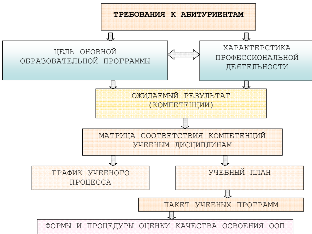
Рисунок 1 - Реализация ООП
