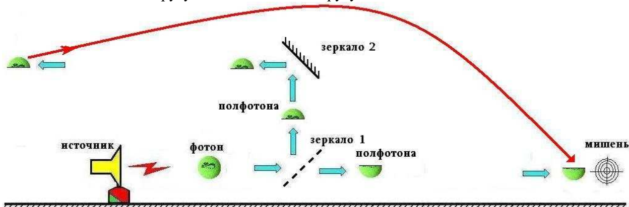
Рис.11. Схлопывание разделенного на половинки фотона
