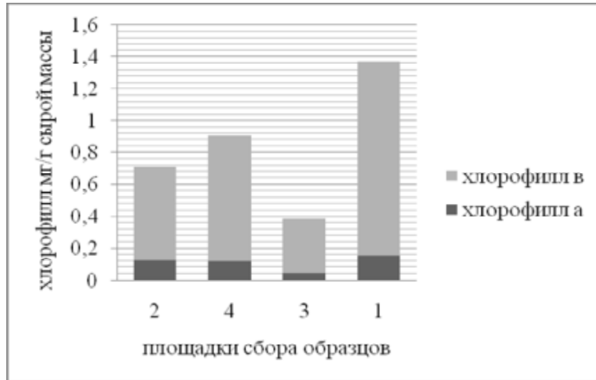
Рис. 2. Содержание хлорофиллов в талломах лишайников Hypogimnia physodes на разных площадках сбора* (по Лихтенталеру), мг/г сырой массы. Площадки: 1- лесная зона в 10 км от города; 3 - 16-й км Самотлорской дороги; 4 - лесная зона в 25 км от города; 2- район «Церковной гривы»
