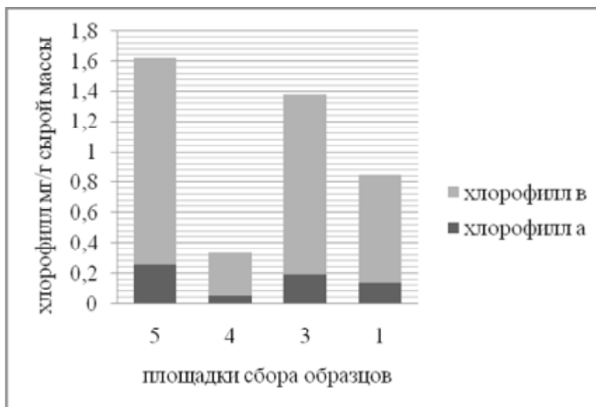
Рис. 1. Содержание хлорофиллов в талломах лишайников Physcia stellaris на разных площадках сбора* (по Лихтенгалеру), мг/г сырой массы. Площадки: 1- лесная зона в 10 км от города; 3 - 16-й км Самотлорской дороги; 4 - лесная зона в 25 км от города, 5- территория городского парка
