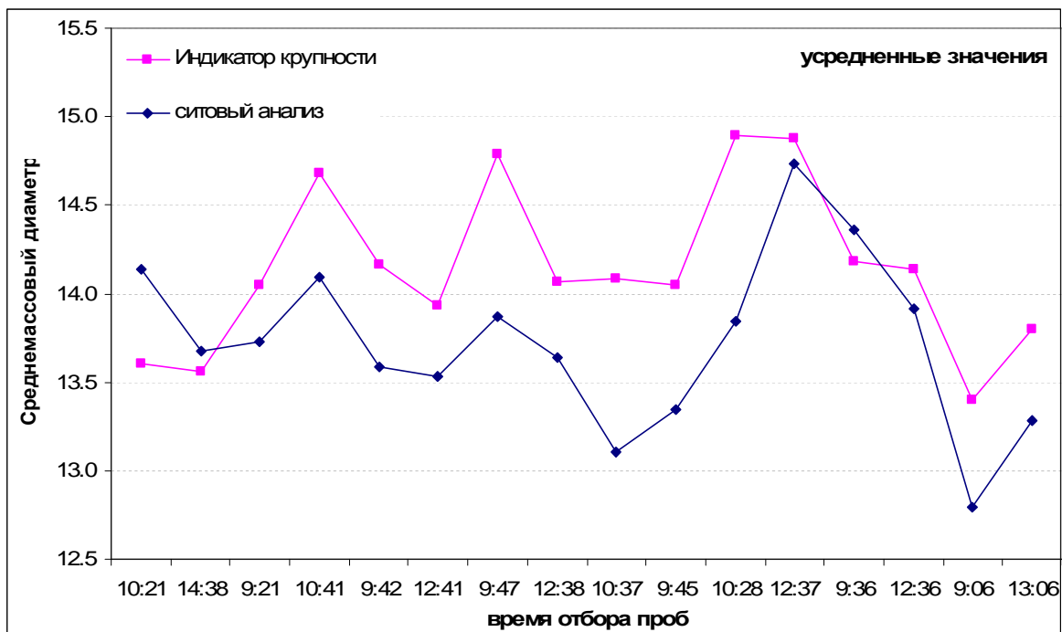
Рис.3. Изменение среднемассового диаметра годных окатышей технологической линии №8 во времени
