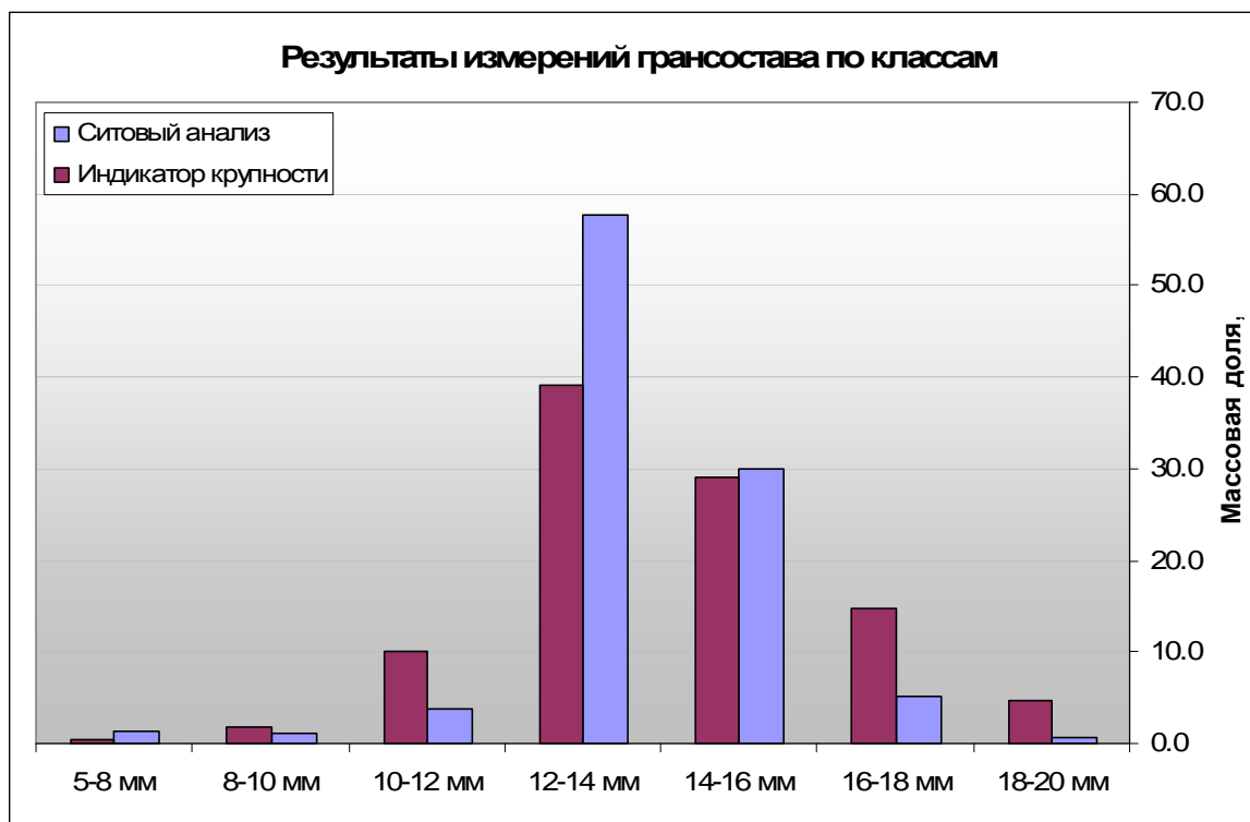
Рис. 2. Результаты тестового определения гранулометрического состава окатышей
