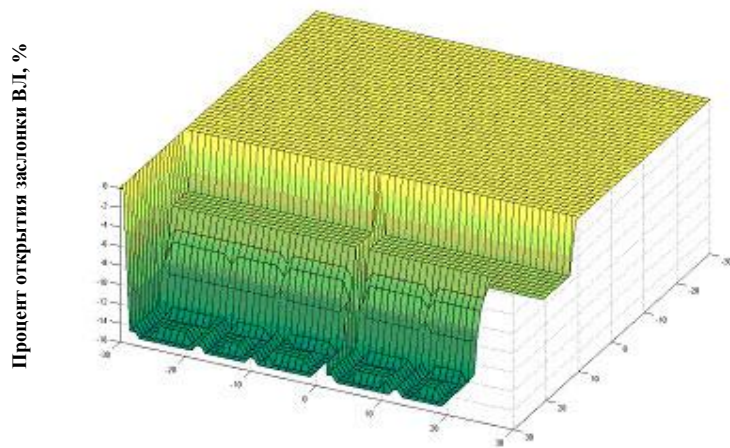
Рис. 9. График зависимости изменения процента открытия заслонки ВЛ от изменения влажности в канале СХ и изменения влажности в канале ВЛ
