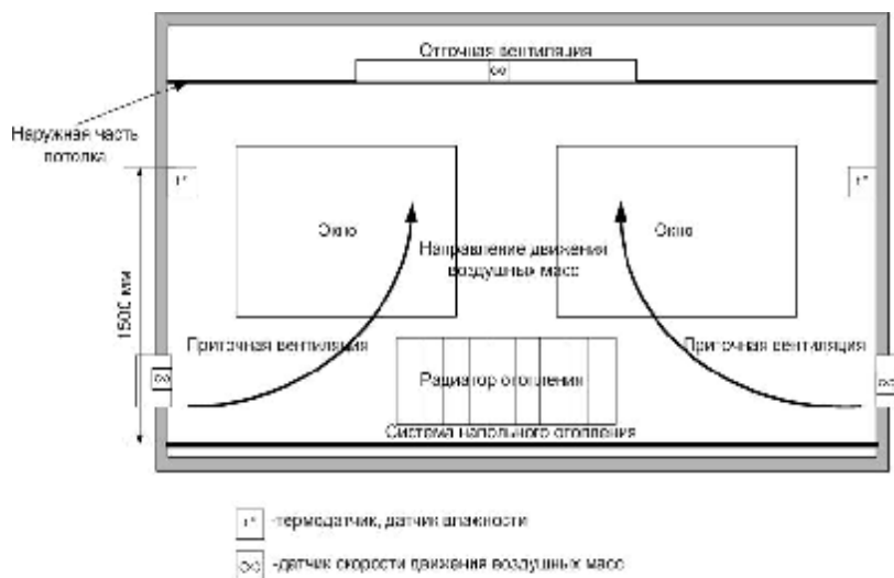
Рис. 1. Помещение в разрезе
