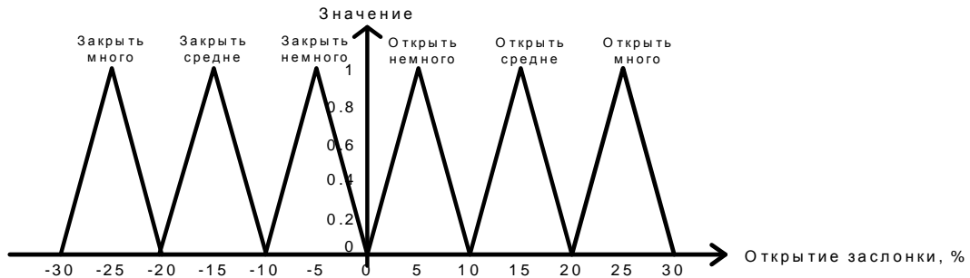
Рис. 5. Графики функций принадлежности для термина лингвистической переменной «процент открытия заслонки СХ»
