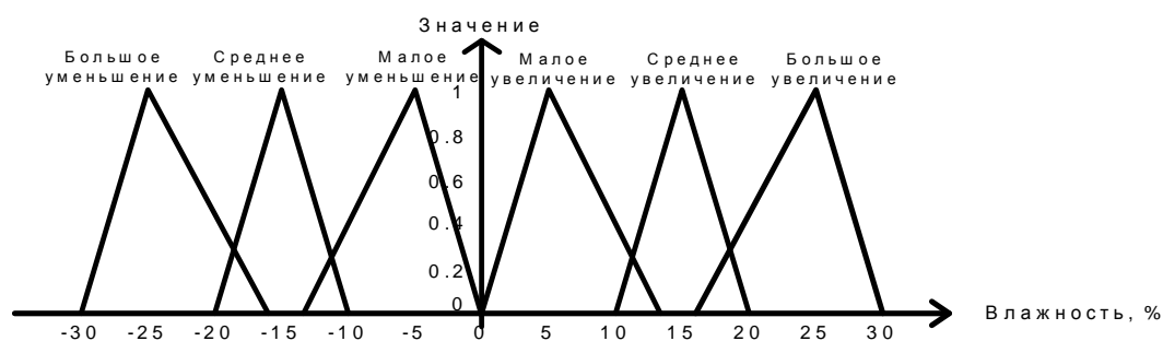
Рис. 3. Графики функций принадлежности для терма лингвистической переменной «изменение влажности в канале СХ»
