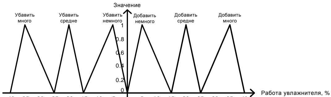
Рис. 7. Графики функций принадлежности для термина лингвистической переменной «процент включения увлажнителя/осушителя»
