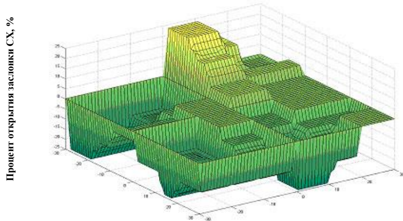
Рис. 8. График зависимости изменения процента открытия заслонки СХ от изменения влажности в канале СХ и изменения влажности в канале ВЛ
