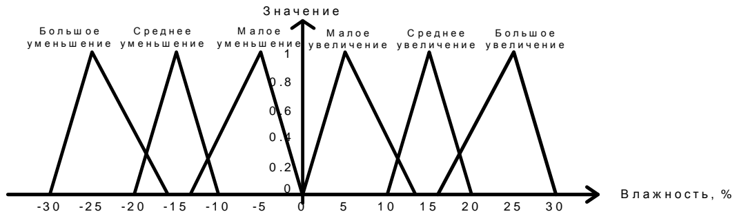
Рис. 4. Графики функций принадлежности для термина лингвистической переменной «изменение влажности в канале ВЛ»
