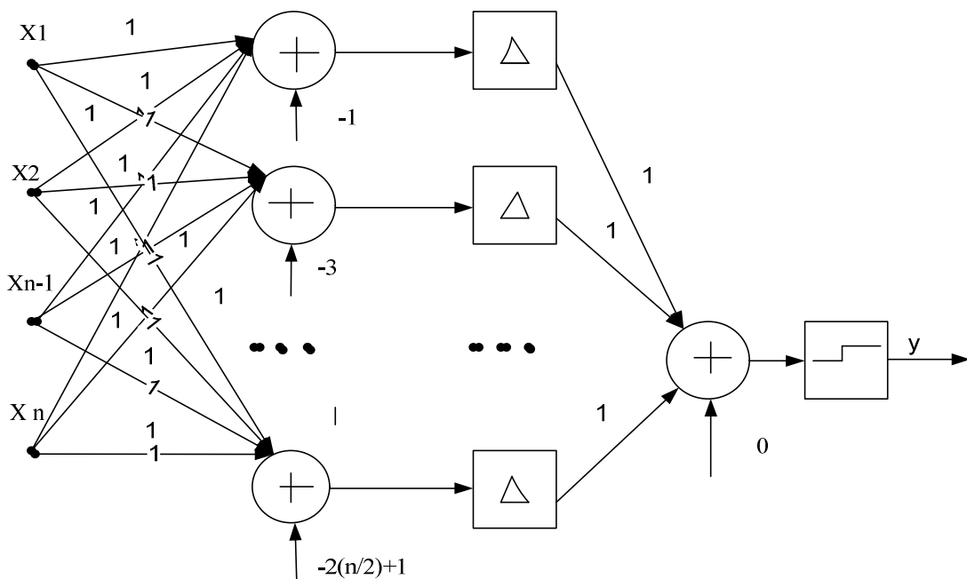
Рисунок 2. Трехслойная нейронная сеть сумматора по модулю два.
