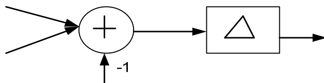
Рисунок 1. Нейросетевая модель двухвходового сумматора по модулю два с использованием треугольной функции активации.
