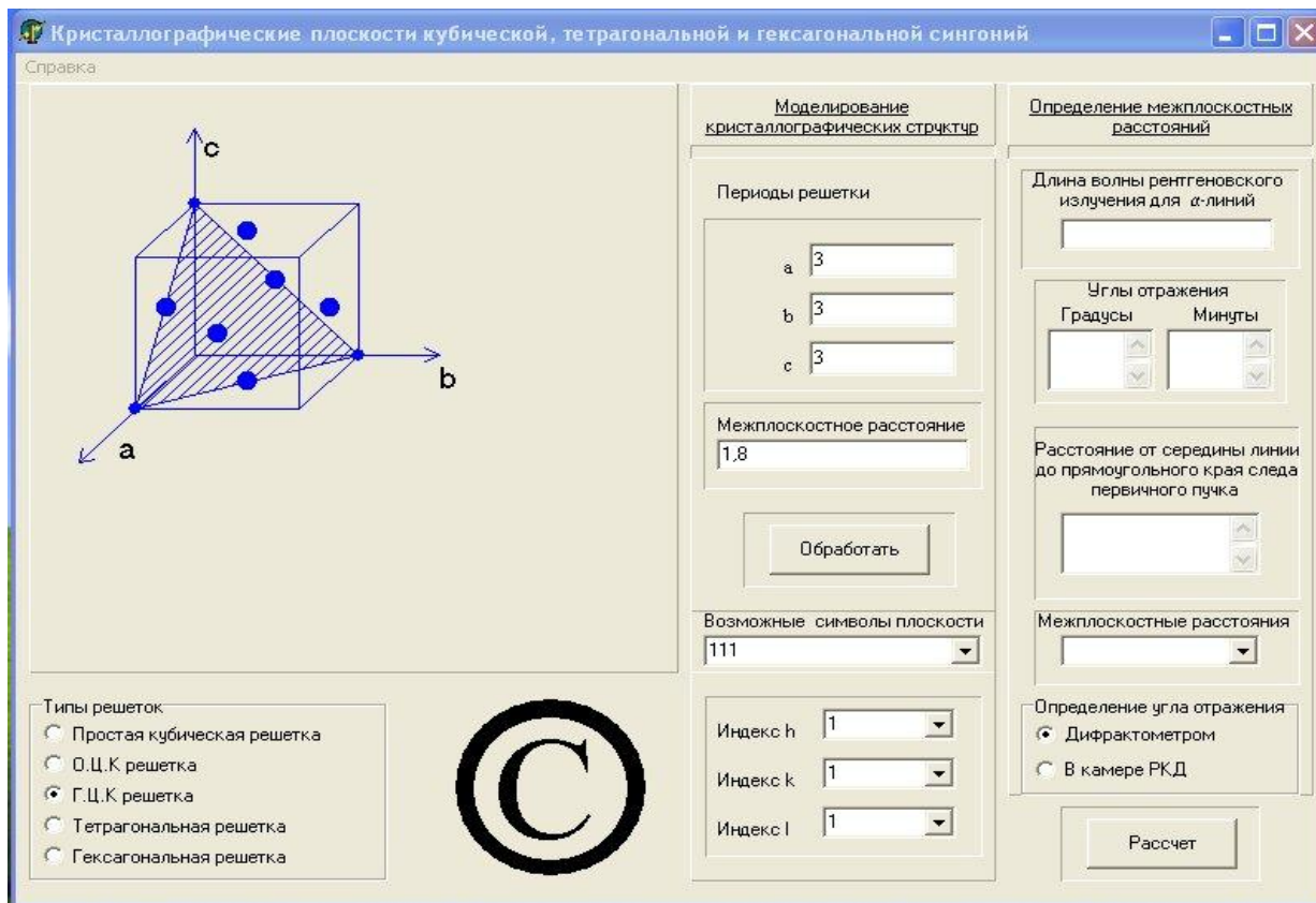
Рис.1.Интерфейс программы.
