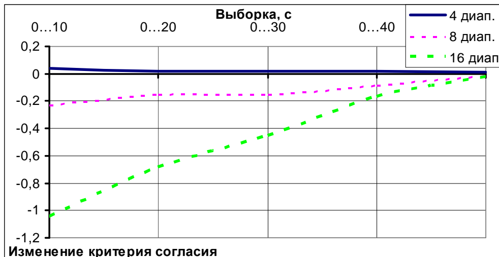
Рис. 2. – Динамика изменения наблюдаемого значения критерия согласия S_2 Пирсона от размера выборки для различного числа диапазонов при уменьшении частоты выборки в десять раз
