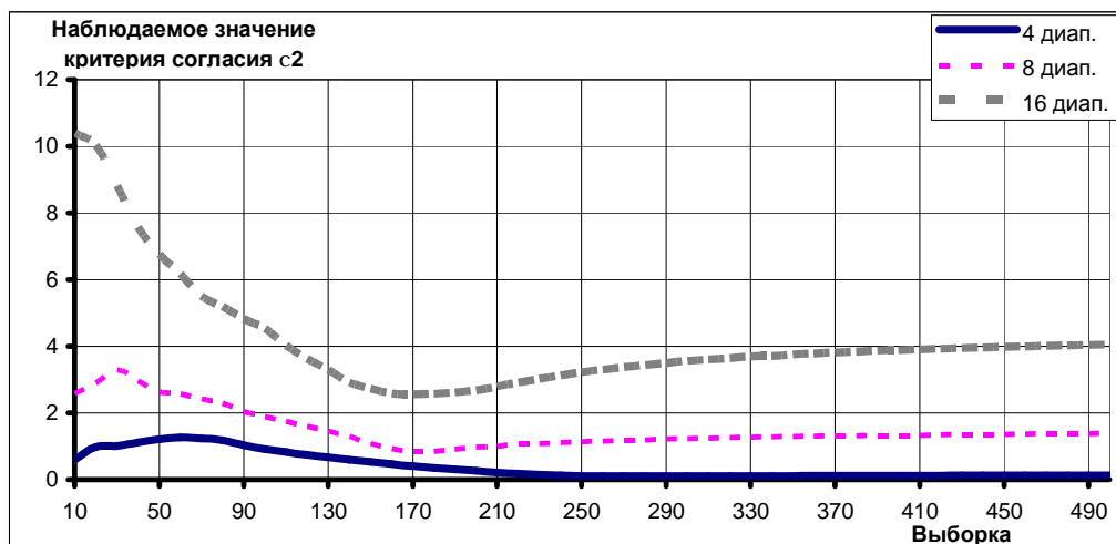
Рис. 1. – Зависимость наблюдаемого значения критерия согласия \chi^2 Пирсона от размера выборки для различного числа диапазонов
