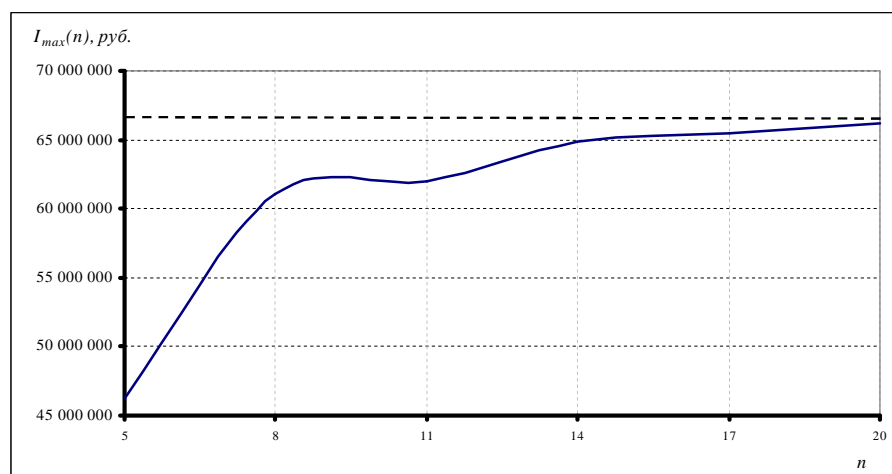
Рис.3. Динамика сходимости максимизированного критерия качества от количества удерживаемых в разложении членов n
