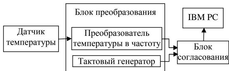
Рис. 2. Структурная схема цифрового термометра
